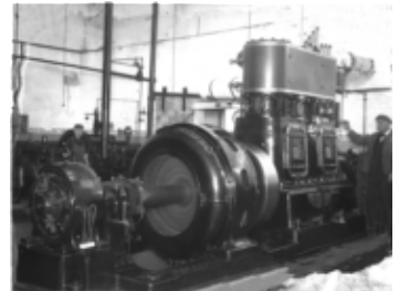
AFC 341-S4-SS1-I14 Generator. -- 1912. -- 6.5x8.5 glass plate negative. -- Box Number AFC 341-4 AFC 341-18
